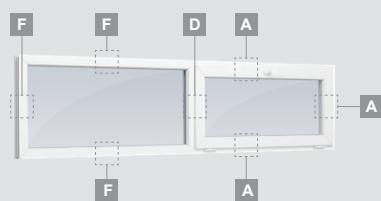
Kaheosaline parempoolse kaldavaneva osaga aken
