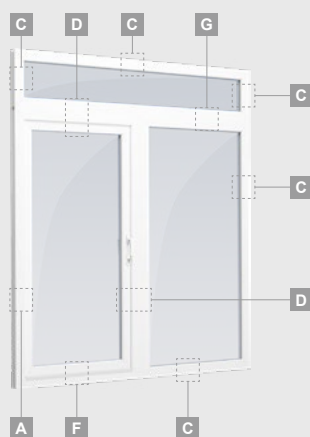
Vitriinaknaga ühendatud ja selle kohal asuva horisontaalse ülaaknaga terrassiüks. Uks asub vasakul
