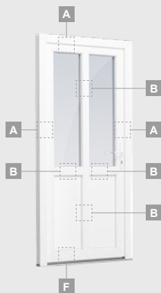
Ühepoolne 1 horisontaalse ja 2 vertikaalse liistuga, 2 PVC-paneeli ja 2 klaasiga välisüks
