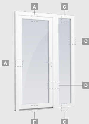
Ühepoolne vitriinaknaga ühendatud välisüks
