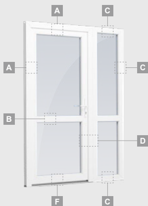
Ühepoolne 2 horisontaalliistu ja klaaspaneeliga vitriinaknaga ühendatud välisüks
