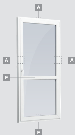
Ühepoolne1 horisontaalliistu ja 2 klaasiga rõduuks
